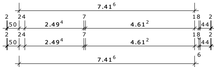
Dachansicht
